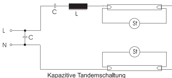
Kapazitive Tandemschaltung
