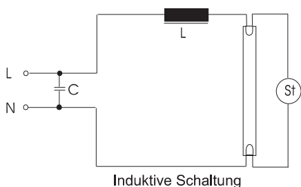
Induktive Schaltung
